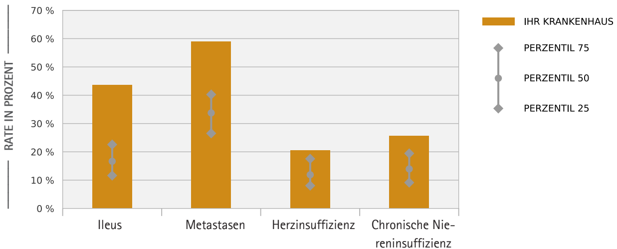
Begleiterkrankungen im Startfall bei Operation bei kolorektalem Karzinom (2019–2021)
